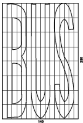
Planche 2. Marques longitudinales provisoires : clous oranges.
